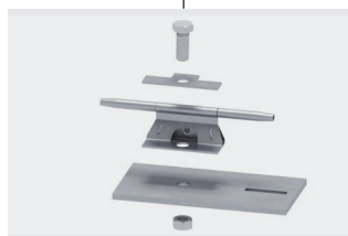
Montaż łącznika pośredniego
