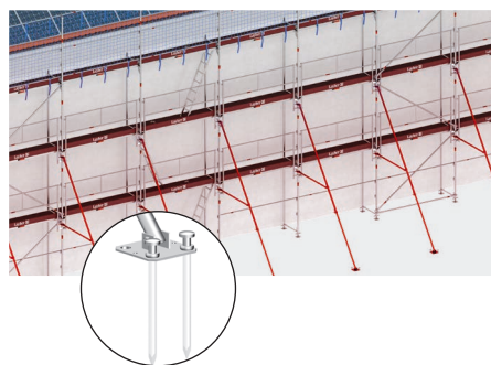
Zaczepek kotwiący, 0.95 m / 1.45 m / 1.75 m, montowane za pomocą dwóch złącz krzyżowych do obu stojaków pionowych.
