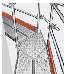
Przykład montażu 45° 9
